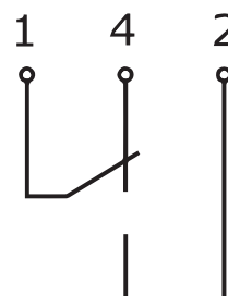
Affectation de raccordement selon EN 50044
