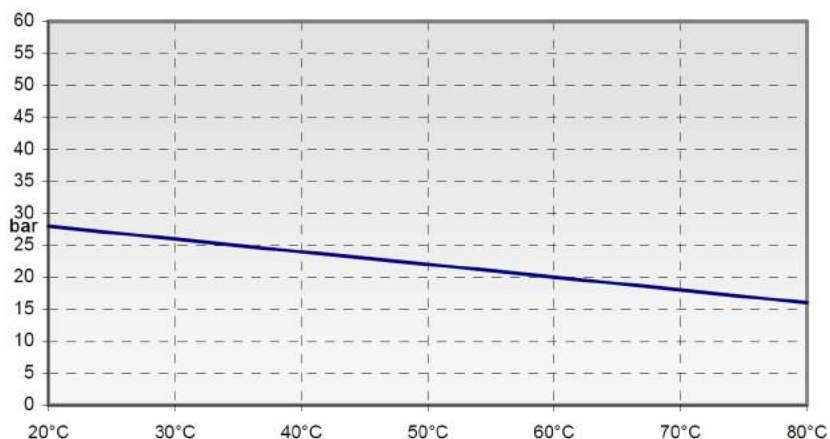
Limite de charge de pression en fonction de la température
