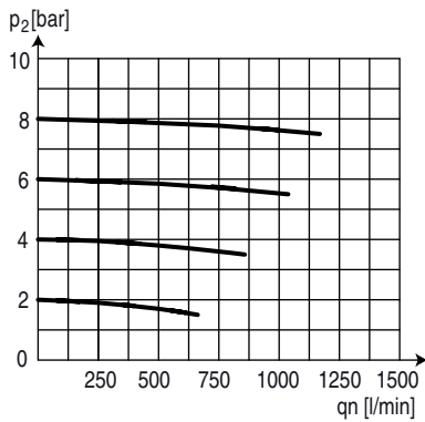
FV.11 Elément filtrant V 23/40
